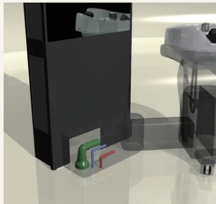
配管カバー内で立ち上げた場合 ※配管カバー床下(EA-YMSPY)をお選びください。
