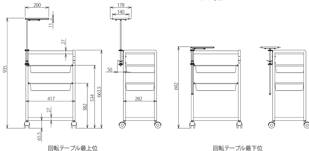
トレイ寸法
